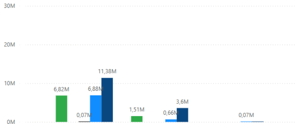
CEPAL
