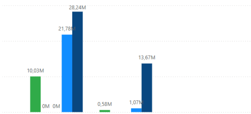
DoValue
